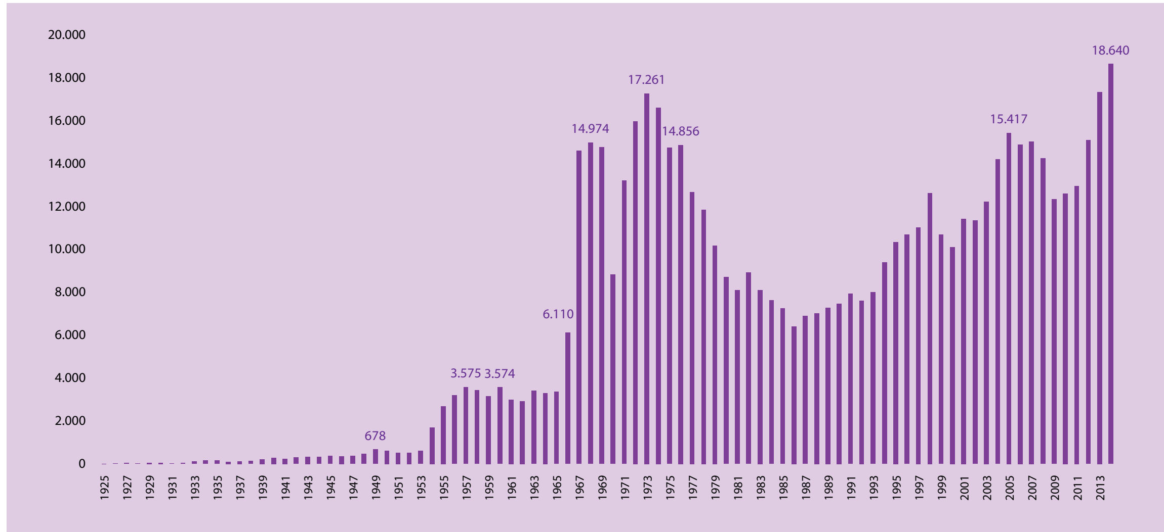
Gráfico N° 12 BOLIVIA: PRODUCCIÓN DE PETRÓLEO Y CONDENSADO, 1925 - 2014 (En miles de barriles)
