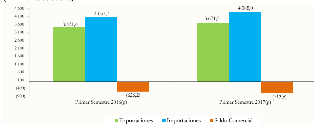
Gráfico N° 1 BOLIVIA: SALDO COMERCIAL, PRIMER SEMESTRE DE 2016 Y 2017 (En millones de dólares)
